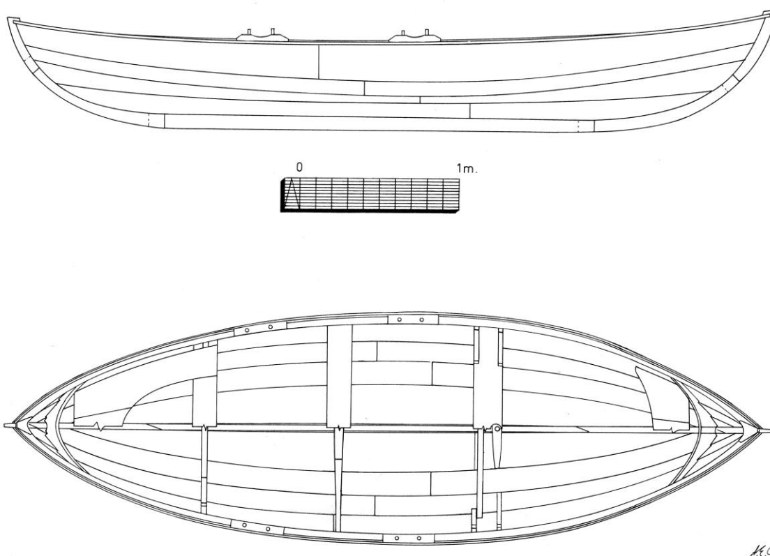
Strandebarmar, oppmålingsteikning av Arne Emil Christensen, Norsk Maritimt Museum.
